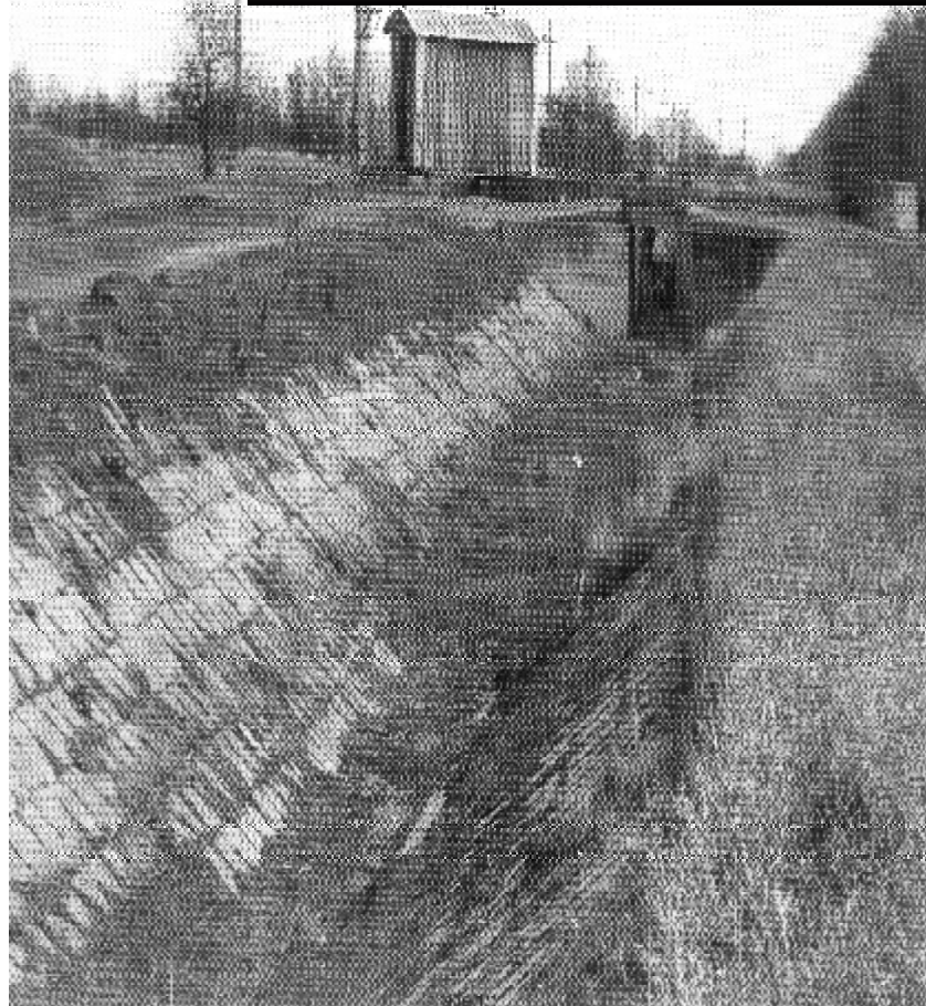
„Consolidare dig Duvalu din incinta Ciuperceni – Desa, județul Dolj”.
